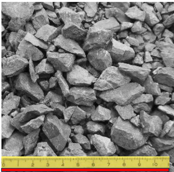
黒クラッシャーラン (粒経 0 ～ 30 mm)
